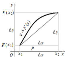
Рисунок 2 - Функция y = F(x) возрастает
