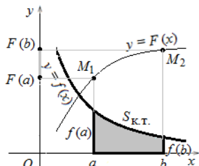
Рисунок 13 - S_{\text{к.т.}} = F(b) - F(a)
