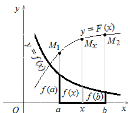
Рисунок 11 - Криволинейная трапеция
