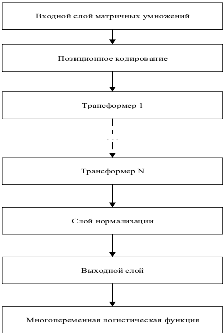
Рисунок 3. Архитектура GPT
