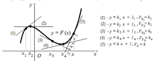
Рисунок 10 - Мгновенная скорость функции y = F(x) в различных точках из области определения
