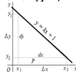
Рисунок 7 - Функция y = kx + l, k < 0
