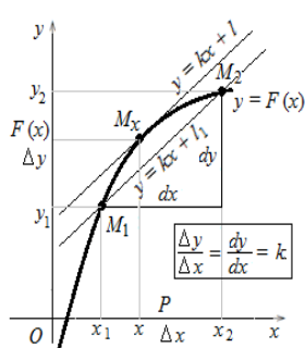
Рисунок 8 - Касательная и секущие Рисунок 9 - Скорость изменения функции
