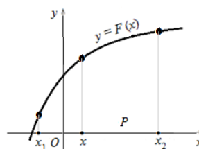
Рисунок 4 - Мгновенная скорость V_{x_1} > V_x > V_{x_2}
