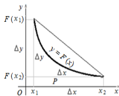
Рисунок 3 - Функция y = F(x) убывает
