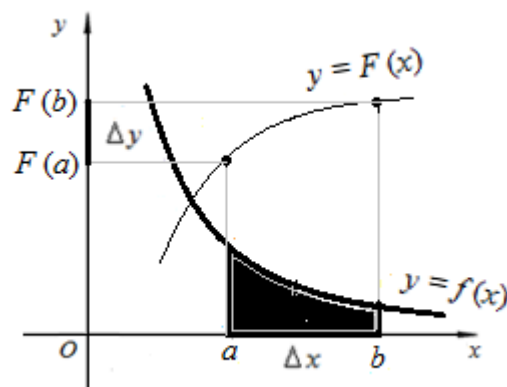
Рисунок 1 - S_{\text{фиг.}} = F(b) - F(a)
