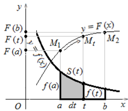
Рисунок 12 - S(t) = F(t) - F(a)
