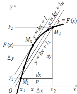
Рисунок 8 - Касательная и секущие Рисунок 9 - Скорость изменения функции
