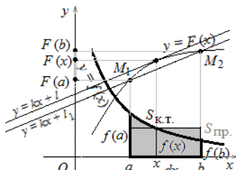
Рисунок 14 - S_{\text{к.т.}} = f(x) \cdot dx
