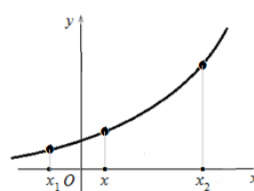
Рисунок 5 - Мгновенная скорость V_{x_1} < V_x < V_{x_2}
