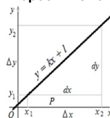
Рисунок 6 - Функция y = kx + l, k > 0
